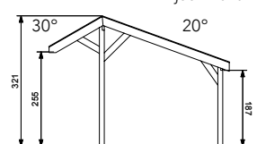
zijanzicht
